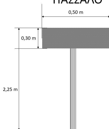
Σκίτσο 13. Εικόνα πλάγιας όψης ξύλινης πινακίδα υποδοχής
