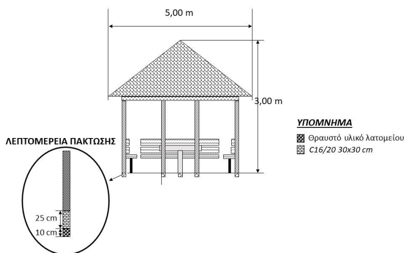
Σκίτσο 4. Εικόνα πρόσοψης ξύλινου κιοσκίου
