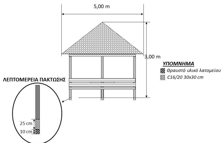
Σκίτσο 6. Εικόνα πλάγιας όψης ξύλινου κιοσκιού
