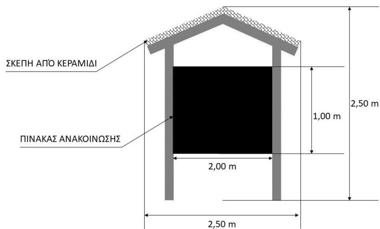
Σκίτσο 10. Εικόνα πρόσοψης ξύλινης πινακίδα υποδοχής
