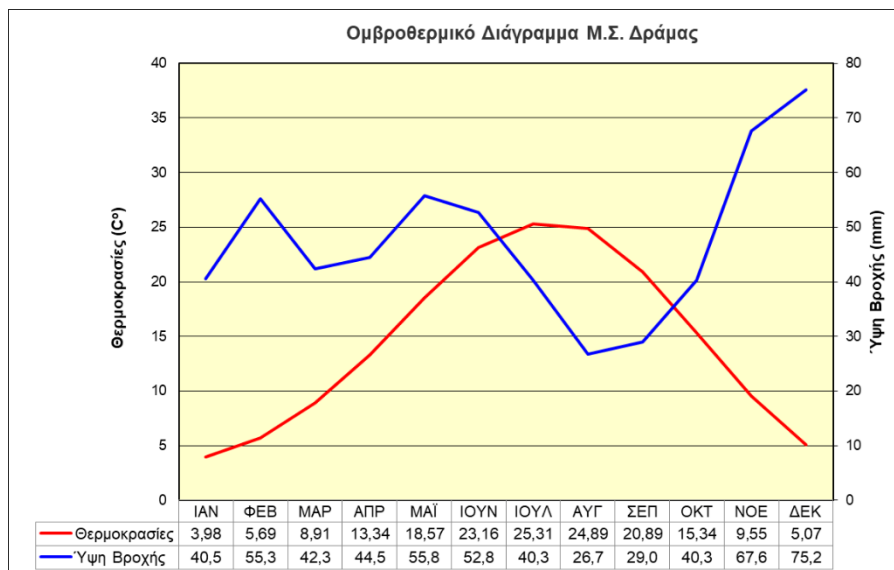
Εικόνα 1 – Ομβροθερμικό διάγραμμα (Bagnouls - Gausson) Μ.Σ. Δράμας.
